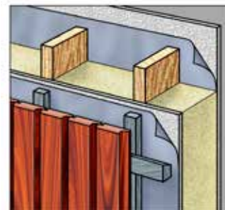
Tekening 7. Een voorbeeld van een dubbel regelwerk.
