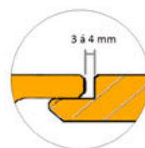
Tekening 9. Voldoende expansieruimte aanhouden tussen delen.
