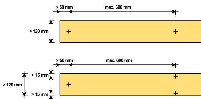
Tekening 8. Maatvoering bevestigingspunten.
