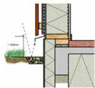
Tekening 10. Bij voldoende afstand tussen hout en maaiveld blijft het hout vrij van opspattend vocht en vuil.
